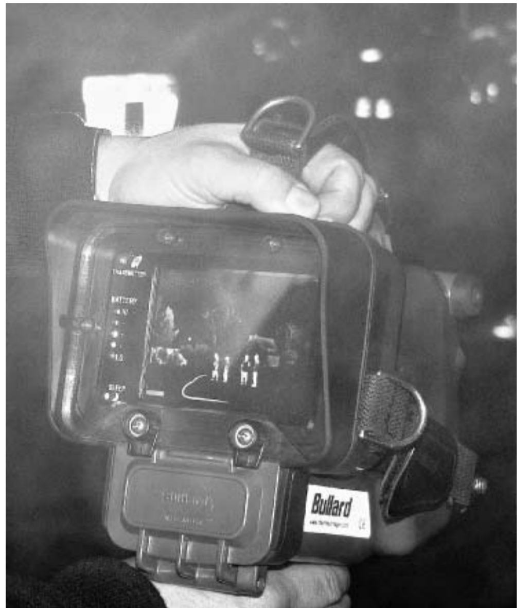
Der Monitor der Wärmebildkamera zeigt überraschend klar und deutlich die Szene. Bei einem Ernstfall können solche Bilder Leben retten.
