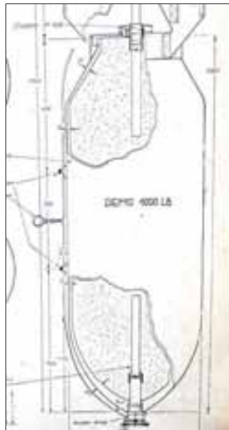
So ist die Bombe aufgebaut.
